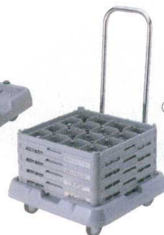
BK ラックドローリー 商品コード ⑦ PR-1 (ハンドル無) 595×595×H182 4973200 ⑧ PR-2 (ハンドル付) 595×595×H940 4973300 材質: 本体/ポリプロピレン樹脂 パイプ/SUS430
