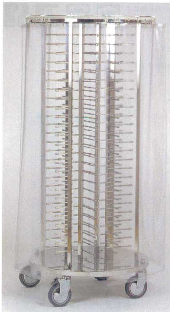
① ディッシュスタック 100 カーテン式 (丸型) EBM 6201100 φ785×H1,790 カバーの取り付け、取りはずしの煩わしさを解消しました。従来の角型から丸型にする事により、全体を均一にカバーします。カーテン式ですので皿の出し入れもスムーズにできます。 ※φ18cm～33cmの皿が使用できます。 ※キャスターφ150 4輪自在 (内2ヶストップバー付)
