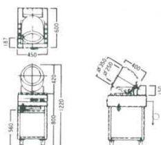
①ロータリーシェフ RC-1 スタンド型 ガス式 外寸：450×600×H1,220
