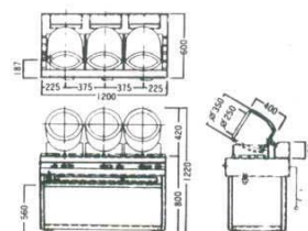
③ロータリーシェフ RC-3 スタンド型 ガス式 外寸：1,200×600×H1,220
