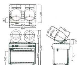
②ロータリーシェフ RC-2 スタンド型 ガス式 外寸：900×600×H1,220
