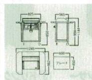
②ステーキテーブル S-116 1244400 キャスター：自在φ100×4（2輪ストッパー付）
