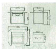
①ステーキテーブル S-111 1244300 キャスター：自在φ100×4（2輪ストッパー付）
