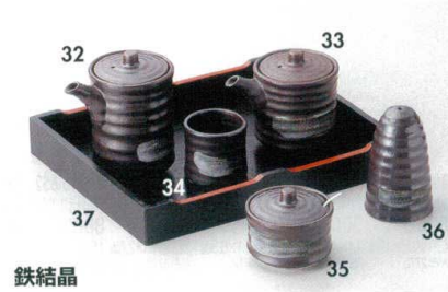
鉄結晶
