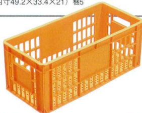
95-20 1-118-7 [P.P] コンテナTP-38 オレンジ ¥3,650 (外寸62.5×29.5×25・ 内寸59.5×26.5×24.2) 梱8
