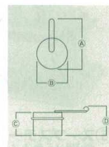
⑨固形用ランプ UK 商品コード (A) (B) (C) (D) 内寸 特大 1490400 320 153 66 85 φ149×H62 大 1490500 219 115 62 75 φ105×H60 中 1490600 206 102 66 83 φ90×H65 小 1490700 186 82 56 70 φ70×H55
