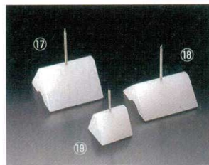
マクラ 活造り用 (2ヶ1組) 商品コード ⑰大 70×65×H90 1573100 ⑱中 70×65×H85 1573200 ⑲小 40×35×H55 1573300 材質: 高圧ポリエチレン ※2個で1組です。
