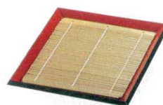
⑫ そば皿 7寸 角型 布目 朱淵黒 外寸：210×210×H30 7537300 材質：本体／ABS樹脂 スダレ／竹製 スダレ：173×173
