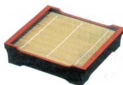
⑭ 盛そばセイロ 角型 貴舟 黒天朱 外寸：200×185×H51 7536500 材質：本体／ABS樹脂 スダレ／竹製 スダレ：172×170
