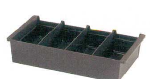
⑥ カトラリーボックス 52652 ヴォルラース 5337800 内寸：250×445×H100 外寸：254×508×H102 材質：ポリプロピレン
