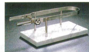
㉓ ハムホルダー 大理石 イタリア 1458300 外寸：600×245×H190 大理石台 480×245 ホルダー 全長：600×H140 最大幅：150 (中心) 最小幅：130 (中心)
