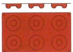
⑦サバラン L (6ヶ取) 2579.28 7385500 出来上り寸法：φ65×H20
