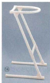
洗面器スタンド イレクター EBM 外寸 商品コード ⑭シングルタイプ 450×440×H750 8380700 ⑮ダブルタイプ 775×335×H750 8380800 ※32cmの洗面器が使用できます。 ※ダブルタイプはキャスター付です。 ※鎖に強く、丈夫で軽い。 ※鋼鉄パイプに樹脂コーティング。
