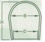
⑤亀ザル 18-8 BK (A) (B) 高さ 商品コード 3升 445 380 145 0422100 ⑩ 5升 480 470 180 0422200 ⑩ 8升 530 520 185 0422300 ⑩ 12升 605 575 200 0422400 ⑤ 全網 0.45×13メッシュ
