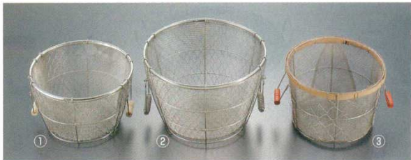
①米揚カゴ 木柄 手付 ステンレス ③米揚カゴ 竹巻 手付 18-8 内寸 商品コード 外寸 商品コード 3升用 φ270×180 0421300 ⑤ 3升用 φ270×190 0421700 1斗用 φ360×230 0421400 ⑥ ※14メッシュ
