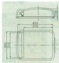
⑧真空包装機 V-381 卓上型 トスパック 7822700 ※ガス封入機能は、オプション (V-381のみ)
