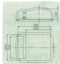
⑦真空包装機 V-281 卓上型 トスパック 7822600
