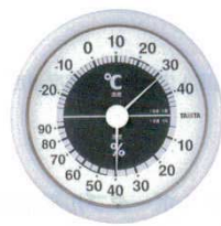
⑤ 温度計 TT-514 ブルー φ182×32 0859300 質量：約230g 測定方式：バイメタル式 表示方法：指針 設置：掛式 測定範囲：温度-20～40℃ (2℃) 湿度10～90% (5%)
