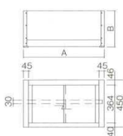
高さ450 (棚板1枚)
