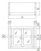
高さ600 (棚板1枚)
