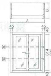
高さ900 (棚板2枚)
