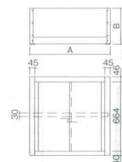
高さ750 (棚板1枚)
