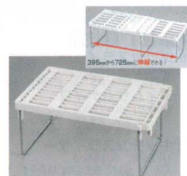
⑬ キッチンラック スライド型 T-115 ㊦ 2913300 外寸：395～725×245×H190 材質：ABS樹脂、鉄クロームメッキ
