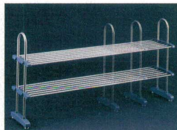
⑧ ワイズスペースラック スライド式 P-2030 約600～1000×230×H525 1132400 ㊦ 材質：フレーム・スライドパイプ/18-8ステンレス 棚枠・棚受/ABS、脚キャップ/エラストマ ●棚は上下左右にスライドしますので、収納物の 高さにあわせて調整できます。 ※幅は600mm～1000mmまで調整可能
