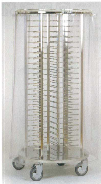
①ディッシュスタック 100 カーテン式 (丸型) EBM 6201100 φ785×H1,790 カバーの取り付け、取りはずしの煩わしさを解消しました。従来の角型から丸型にする事により、全体を均一にカバーします。カーテン式ですので皿の出し入れもスムーズにできます。 ※φ18cm～33cmの皿が使用できます。 ※キャスターφ150 4輪自在 (内2 ケストッパー付)
