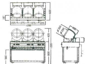
③ロータリーシェフ RC-3 スタンド型 ガス式 外寸：1,200×600×H1,220
