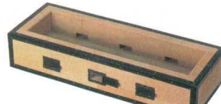
④バーベキューコンロ BQ22号 炭用 6559700 外寸：930×350×H210 内寸：800×215×H115 重量：25kg 付属品：焼きアミ
