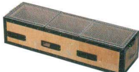
②バーベキューコンロ BQ8T号 炭用 6559600 外寸：770×230×H200 内寸：690×150×H110 重量：17kg 付属品：焼きアミ
