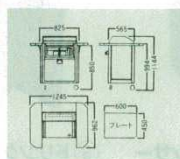
②ステーキテーブル S-116 SS 1244400 キャスター：自在φ100×4（2輪ストッパー付）
