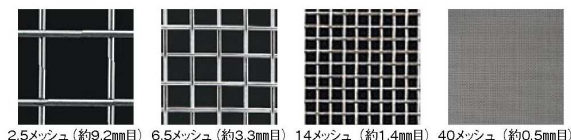
2.5メッシュ (約9.2mm目) 6.5メッシュ (約3.3mm目) 14メッシュ (約1.4mm目) 40メッシュ (約0.5mm目)
