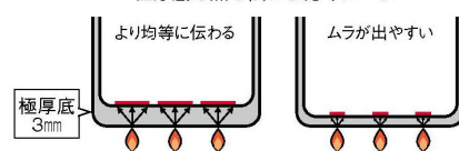
極厚底の熱の伝わり方イメージ
