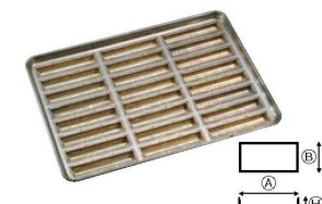
⑮シリコン加工 ラフト型 天板 (24ヶ取) 5396000 ¥24,600 外寸:545×395×H38 単品寸法: A150 B26 H18
