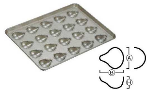
⑥シリコン加工 ビュアベル型 天板 (20ヶ取) 6739800 ¥21,600 外寸:545×395×H57 単品寸法: A65 B74 H36
