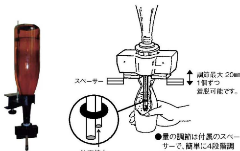
② フンシヨットメジャーマルチⅡ クランプタイプ ロングマルチ 72 4923810 ¥14,000 本体外寸:110×140×H605 ●標準タイプより70mm長い120mmのロングノズル仕様 ●ノズルの先端に液体が触れると注入が止まる為、長さのあるグラスで少量必要な場合に適しています。 ●焼酎の水割等に最適です。
