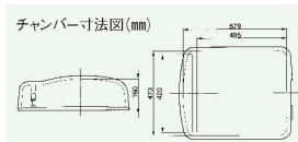
②卓上型 真空包装機 V-482 7811810 ¥977,000
