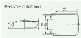
③卓上型 真空包装機 V-380G (ガス封入機能付) 7811700 ¥626,000
