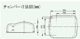
④卓上型 真空包装機 V-280A 7811500 ¥418,000
