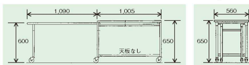
⑰18-8 給食配膳台 2連
