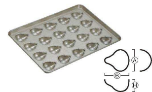
⑥シリコン加工 ピュアペル型 天板 (20ヶ取) 6739800 ¥21,600 外寸:545×395×H57 単品寸法: A65 B74 H36
