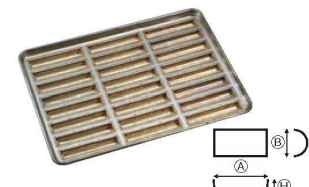
⑮シリコン加工 ラフト型 天板 (24ヶ取) 5396000 ¥24,600 外寸:545×395×H38 単品寸法: A150 B26 H18
