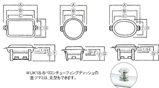
②UK 18-8 バロン 角 チューフィンディッシュ ダブル ※フードパン(上皿)のみダブル仕切ですが、蓋はシングル カバーになります。 ※20インチのみダブルカバーもあります。
