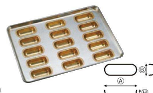
⑭シリコン加工 フィンガー型 天板 (15ヶ取) 外寸 商品コード 価格 L 545×395×H57 5395800 ¥22,000 M 545×395×H55 5395900 ¥21,000 単品寸法: L A116 B49 H35 M A103 B46 H33
