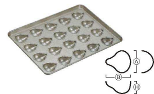
⑥シリコン加工 ピュアペル型 天板 (20ヶ取) 6739800 ¥22,000 外寸:545×395×H57 単品寸法: A65 B74 H36
