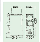
⑨酒燗器 Ti-2 0811200 ¥95,000 電源:100V 消費電力:500W
