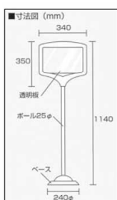
■寸法図 (mm)
