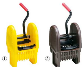
ラバーメイド ブルートモップリンガー (ダウンプレッシャータイプ) 中型 7575-88 ¥33,200 ①イエロー 5332010 ②ブラウン 5332110 342×335×H685 材質:本体/ポリエチレン ハンドル/スチール ※許容モップ幅:210mm
