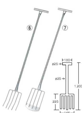
⑥ EBM 18-8 共柄 給食用 熊手フォーク 8203100 ¥13,200 重量:1.2kg
