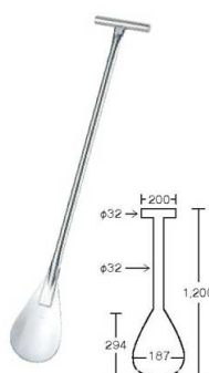
③ EBM 18-0 共柄 特大ヘラ型 給食用 シャモジ 8202500 ¥14,800 重量:2.0kg
