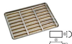
⑮シリコン加工 ラフト型 天板 (24ヶ取) 5396000 ¥25,000 外寸:545×395×H38 単品寸法: A150 B26 H18
