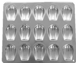
①ギルア マドレーヌ型 マドレーヌシェール型 15ヶ取 No.909 6621500 ¥1,400 外寸:270×228×H13 (1ヶ当り40×56×H12) 材質:スチール・クロームメッキ
