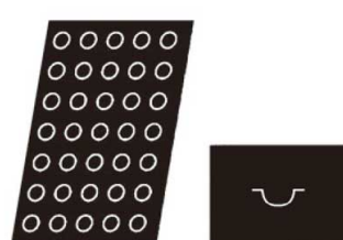
⑪ 1265 ブティフル (半球) ㊦ 5437000 ¥14,500 フレキシパンサイズ: 400×300 8枚取サイズ 出来上がり寸法: φ29 × H18 配列: 7×5 35ヶ取
