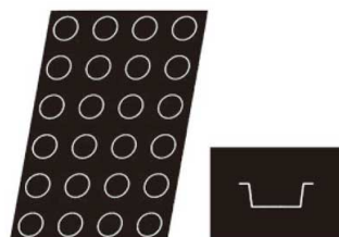
⑤ 2269 パヴァロワ (円柱) ㊦ 6958300 ¥25,000 フレキシパンサイズ: 600×400 フレンチサイズ 出来上がり寸法: φ63 (φ53) × H25 配列: 6×4 24ヶ取
