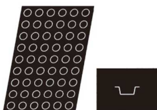
② 1129 ブティフル (円) ㊦ 6205200 ¥25,000 フレキシパンサイズ: 600×400 フレンチサイズ 出来上がり寸法: φ40 (φ33) × H20 配列: 9×6 54ヶ取
