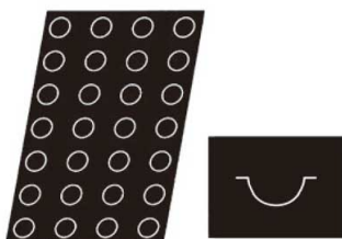
⑨ 1896 ブティガトー (半球) ㊦ 6205500 ¥25,000 フレキシパンサイズ: 600×400 フレンチサイズ 出来上がり寸法: φ58 × H31 配列: 7×4 28ヶ取
