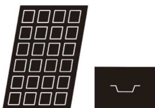
⑫ 1544 フィナンシェ (正方形) ㊦ 5436900 ¥23,000 フレキシパンサイズ: 500×400 6枚取サイズ 出来上がり寸法: 60×60 (33×33) × H15 配列: 4×6 24ヶ取
