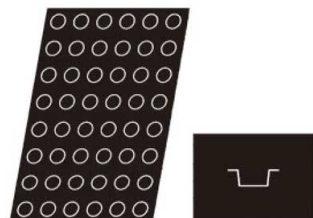
① 2266 ブティフル (円) ㊦ 6205300 ¥25,000 フレキシパンサイズ: 600×400 フレンチサイズ 出来上がり寸法: φ40 (φ33) × H20 配列: 8×6 48ヶ取
