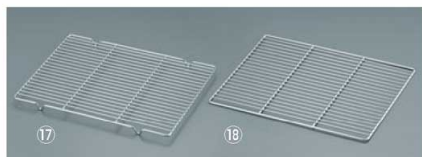
EBM 18-8 ケーキクーラー 角型 外寸 ⑬足付 価格 ⑭足無 価格 大 600×400 1490800 ¥4,600 1491100 ¥4,600 中 500×350 1490900 ¥3,800 1491200 ¥3,800 小 400×300 1491000 ¥3,200 1491300 ¥3,200 目の間隔:11mm 足付の高さ:20mm
