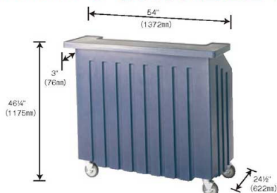
① キャンブロ ポータブルカムバー BAR540
