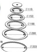
①角カマド AK-41
