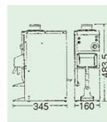
⑦酒燗器 Ti-1 ㉔ 0811100 ¥90,000 電源:100V 消費電力:500W
