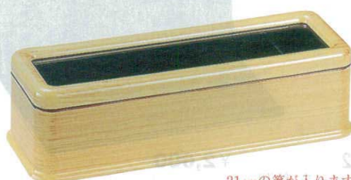
21cmの箸が入ります。 6-1427-3 ¥4,300 白木刷毛目塗 (楊枝入付) [A] 280×105×85 5-1210-3 (82013560)
