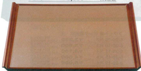
奥広フライト盆 銀透き潤べつ甲SL [A] ノンスリップ加工 6-21-13 尺3 ¥3,600 394×310×19 5-13-13 (15003520) 6-21-14 尺4 ¥4,100 425×340×20 5-13-14 (15003530) 6-21-15 尺5 ¥4,650 456×355×21 5-13-15 (15003540)
