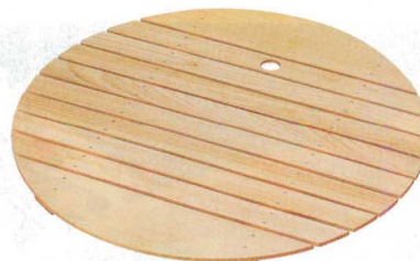
こね鉢盛器用 木製目皿 [木] 6-526-5 尺6寸用 ¥9,000 φ407×65 5-440-5 (45022267) 6-526-6 尺8寸用 ¥9,500 φ470×65 5-440-6 (45022271)
