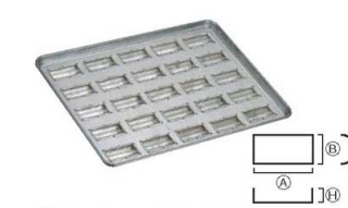
⑫シリコン加工 半円筒型天板 (25ヶ取) 6738900 ¥27,000 外寸:545×395×H40 単品寸法: A75 B32 H18
