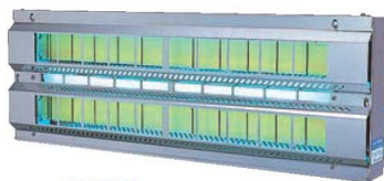
屋内用 ④ピオニー 捕虫器 ㍿ ページコード 商品コード 価格 F-200X型 1-2090-0401 4397000 ¥34,800 716×97×H236 重量:2.6kg(捕虫ランプ含む) 電源:単相100V 有効面積:40~60㎡ 誘虫ランプ:20W×1灯(FL-20SBL) 本体:18-8ステンレス製、インバーター方式 捕虫テープ2枚入り ※吊下げ、壁掛けタイプ ●害虫を落とすので、手でキャッチし、捕虫テープの取り替えだけで、死がいの処理がワンタッチで衛生的です。 捕虫テープ(20枚入り) 1-2090-0402 4265400 ¥6,000 ㍿
