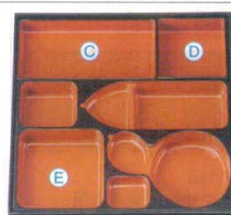
⑩ [A] 8.5寸松花堂用 1-334-8 A仕切 朱天黒 C ¥850 (23.4×11.7×4.1) 1-358-4 [A] 華角鉢 朱天黒 D ¥600 (11.8×11.8×4.4) 1-272-6 [A] 尺3寸長手松花堂用 D.X仕切 朱天黒 E ¥1,850 (35.2×23.5×4.2)
