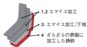
黒マットエマイユ加工の構造
