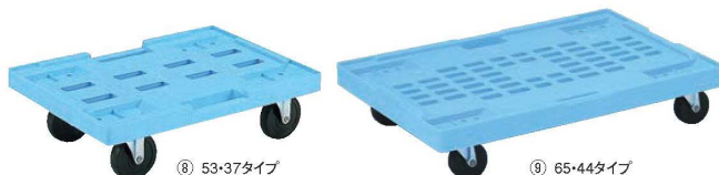
⑧ 53・37タイプ 加 RS折りコン キャリー ページコード 外寸 高さ 商品コード 価格 (8)53・37タイプ 2-0719-0801 534×370 160 3654700 ¥13,500 キャスター:4インチエラストマー車 30ℓ・50ℓ用(①②③④⑤に対応) (9)65・44タイプ 2-0719-0901 650×440 134 3654800 ¥17,680 キャスター:3インチエラストマー車 75ℓ用(③④⑤に対応) 材質:ポリプロピレン 重量:3.1kg
